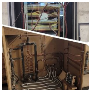
Plomberie - chauffage →
