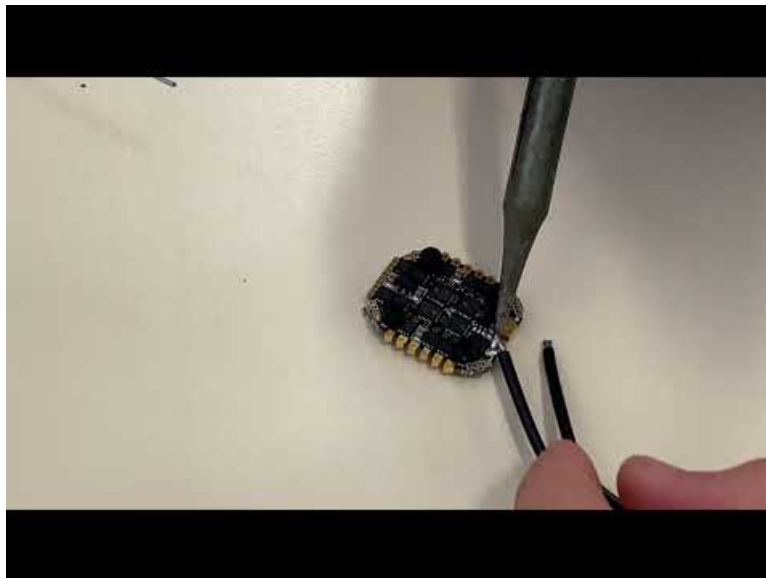
Soudure des câbles de l'accu sur le contrôleur (Video Youtube)
